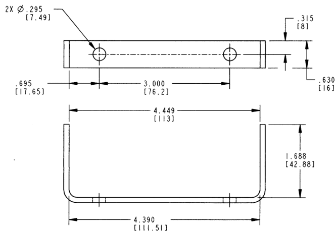
安装支架
